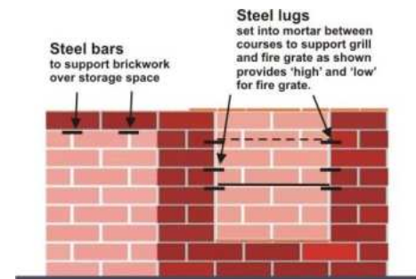
SECTION D-D
